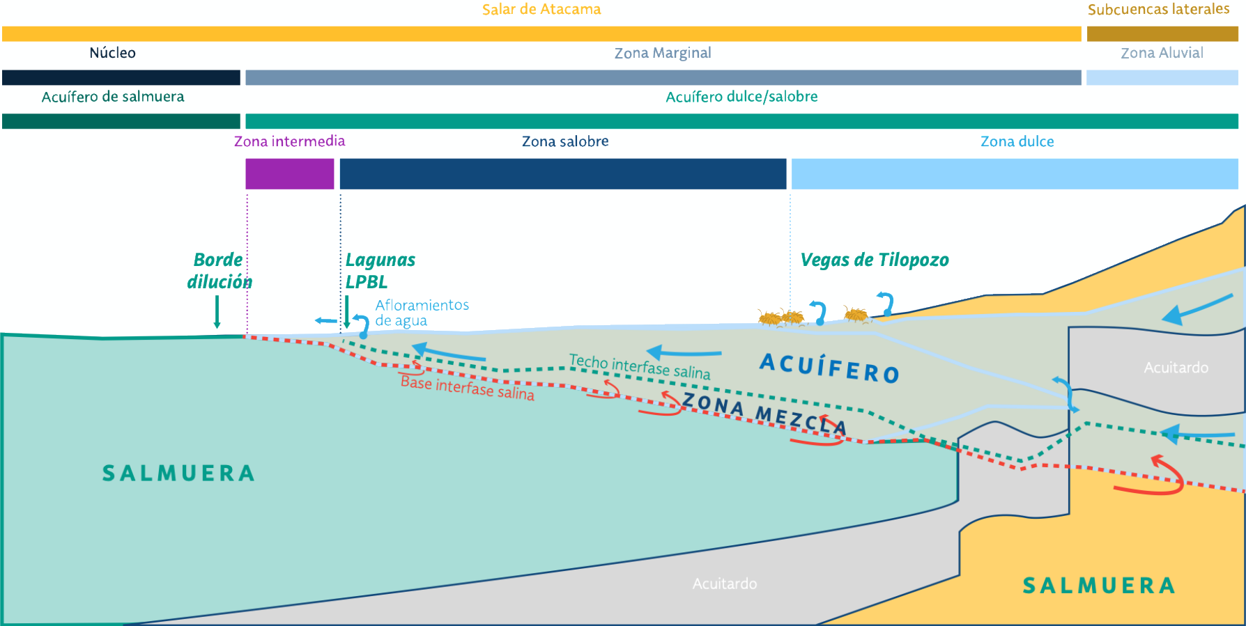
Esquema conceptual de la interfase salina en Zona Marginal Sector La Punta La Brava, 4ª actualización de modelo Albemarle
